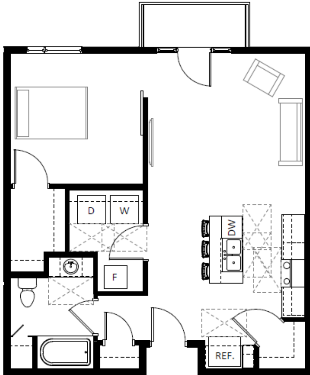
1 1 B.R. UNIT - 1C - 728 SF SCALE: 1/4" = 1'-0"
