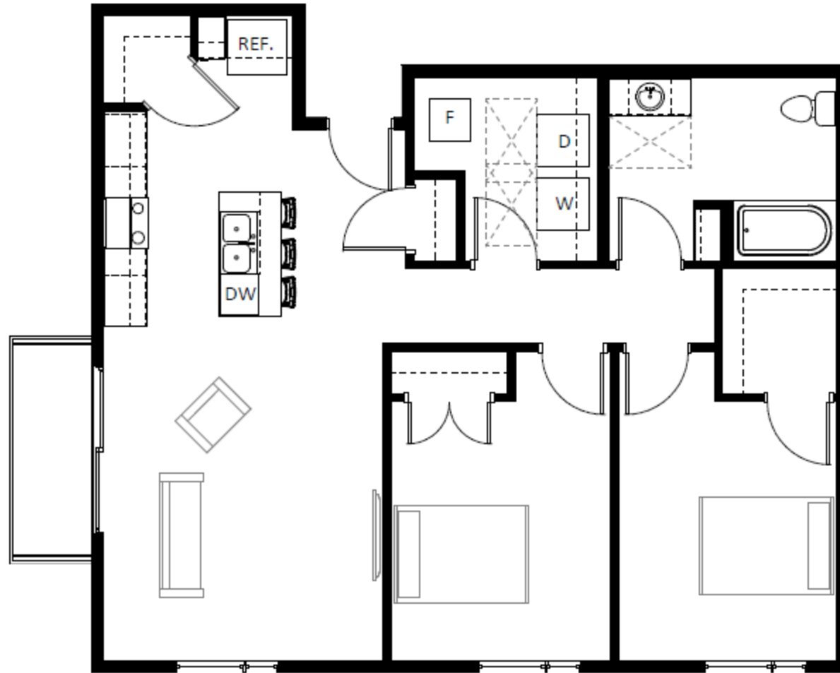
1 2 B.R. UNIT - 2B - 1,009 SF SCALE: 1/4" = 1'-0"
