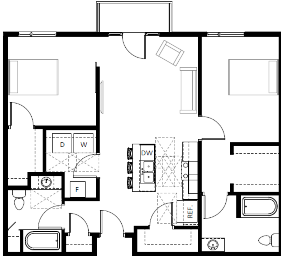
1 2 B.R. UNIT - 2A - 983 SF SCALE: 1/4" = 1'-0"
