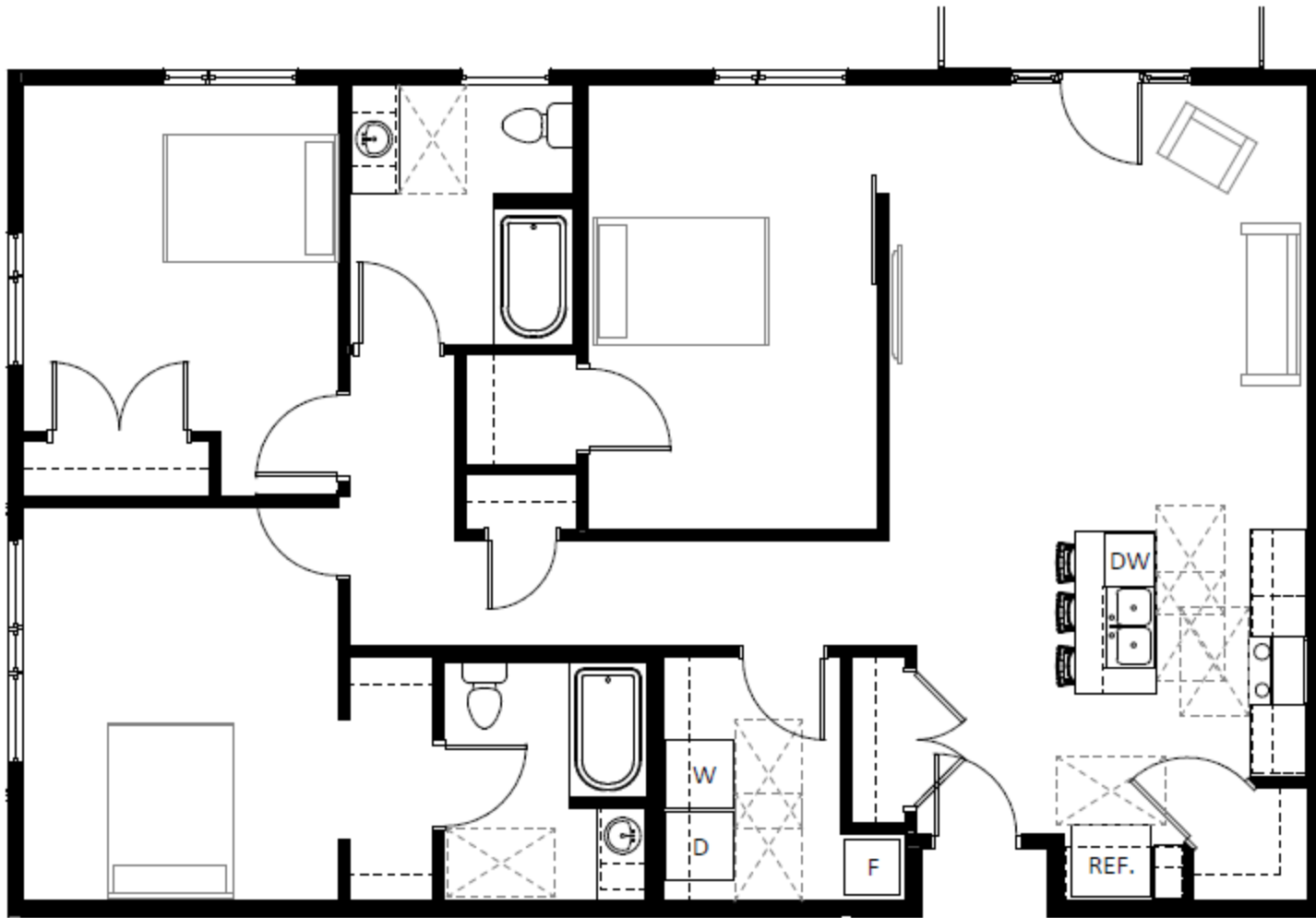
1 3 B.R. UNIT - 3A - 1,417 SF SCALE: 1/4" = 1'-0"
